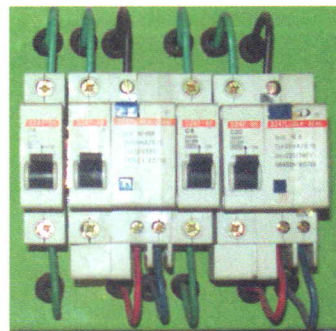
图 9-2-9 家庭配电箱中的空气开关和漏电保护器
