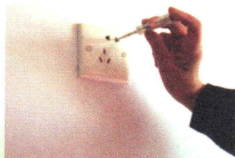
图 9-1-8 用验电笔检验插座的相线
