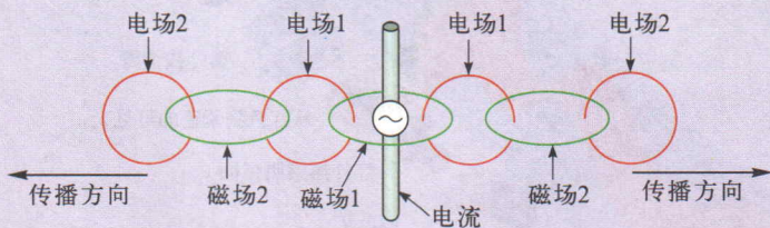
图 10-1-8 电磁波的产生
