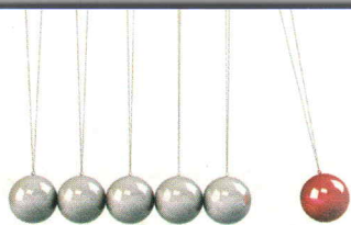
图 11-1-1 摆球的碰撞
