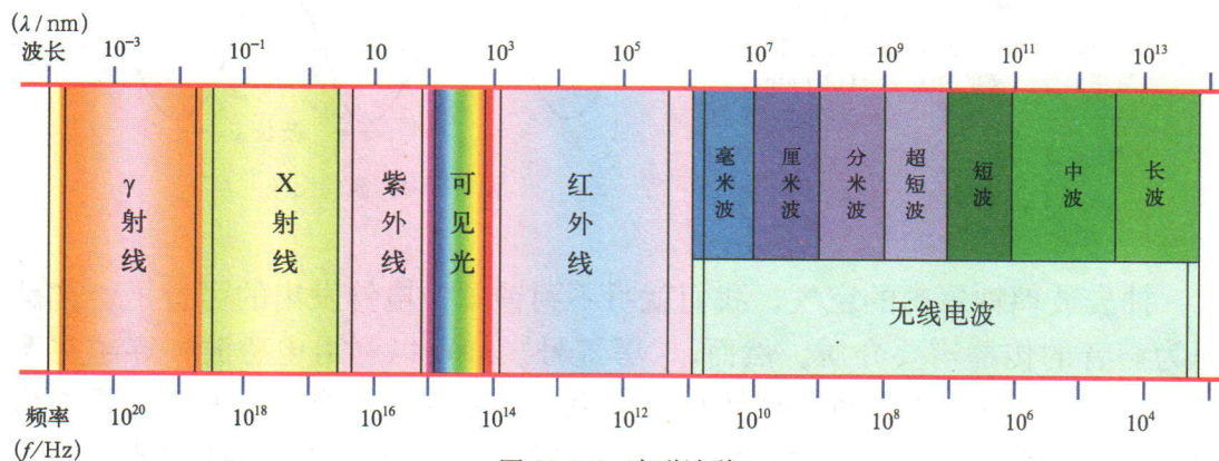
图 10-1-6 电磁波谱
