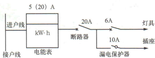
图 9-2-13 多回路配电线路
