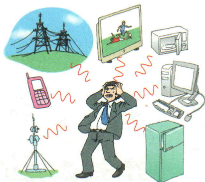
图 10-2-8 电磁波的海洋
