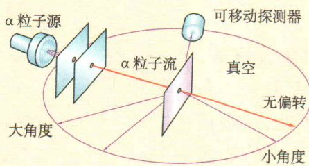
图 11-4-9 \alpha 粒子散射实验装置示意图。实验发现, 大多数 \alpha 粒子都能自由地穿过金箔, 少数 \alpha 粒子发生一个角度很小的偏离, 偶尔能观察到大角度散射。由此, 卢瑟福确认, 原子内部只有非常小的空间集中了能对 \alpha 粒子发生碰撞的物质, 原子内绝大部分空间是空虚的
