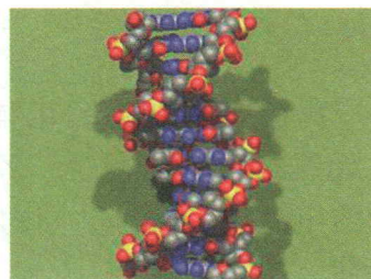
(c) 利用 X 射线可以进行晶体的微观结构研究。在 DNA 双螺旋结构的发现中, X 射线起到了重要作用
