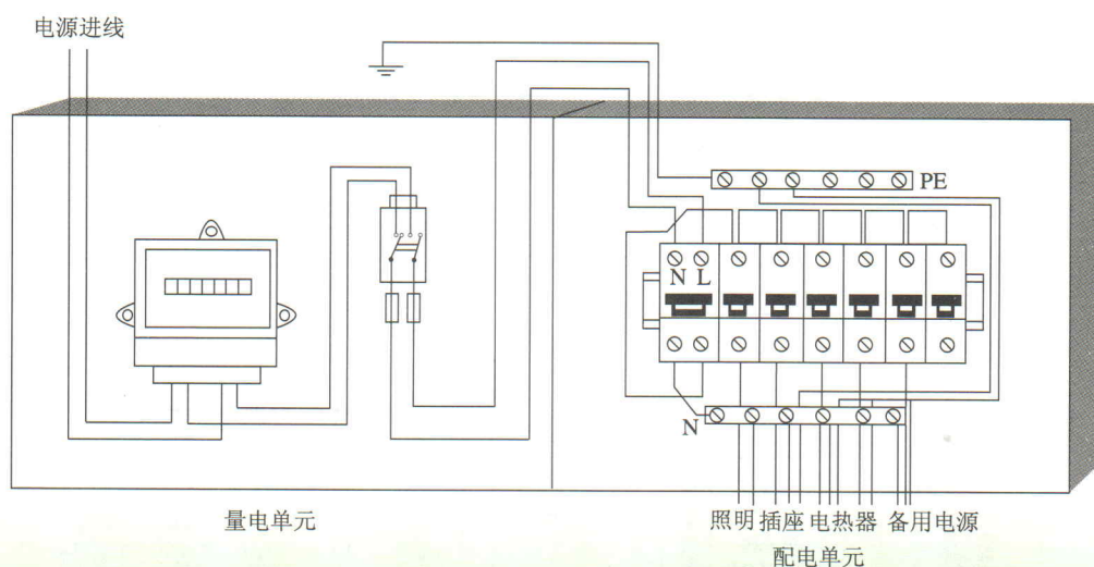
图 9-2-3 家庭电路的量电装置和配电装置
