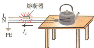
图 9-3-7 有保护接地,发生相线与用电器金属外壳连通故障时,故障电流会使熔断器熔断或使断路器、漏电保护器自动切断电源
