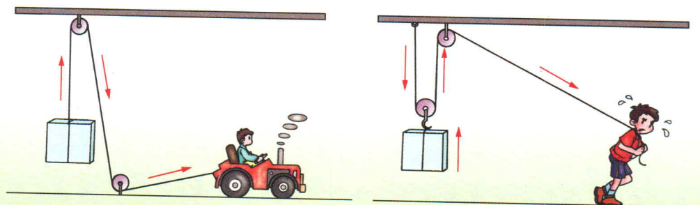
图 11-2-7 滑轮的组合
