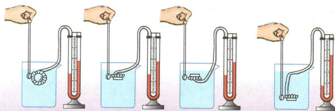
图 9-2-3 探究液体内部压强的规律
