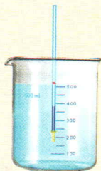
图 10-4-13 简易密度计
