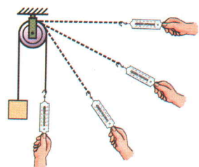
图 11-2-3 定滑轮
