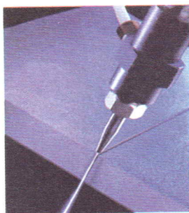
(b) 切割大理石、钢板的“水刀”可对切割表面产生高达 10^8 \sim 10^9 \text{ Pa} 的压强
