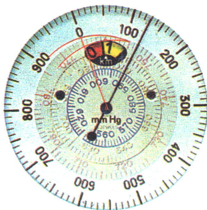
图8-32 无液气压计
