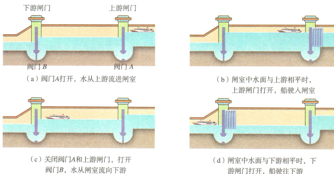
图8-22 船只从上游驶往下游时闸门的开闭情况
