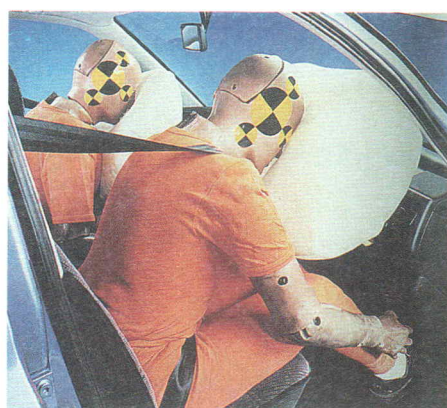
图7-33 采用安全带及安全气囊防护的模拟碰撞实验
