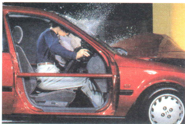
图7-32 未使用安全带防护措施的模拟碰撞实验
