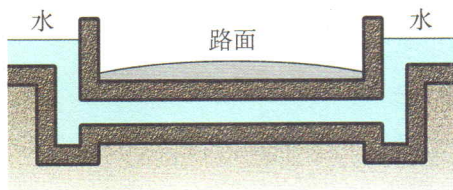
(b) 过路涵洞
