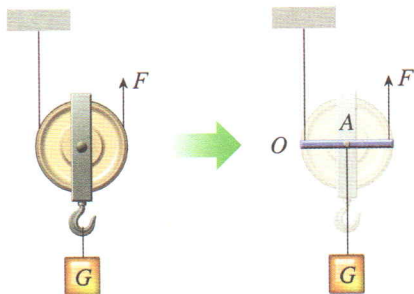
图6-57 对动滑轮作用的分析
