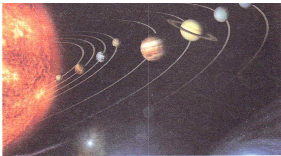
图7-6 八颗行星围绕着太阳运动
