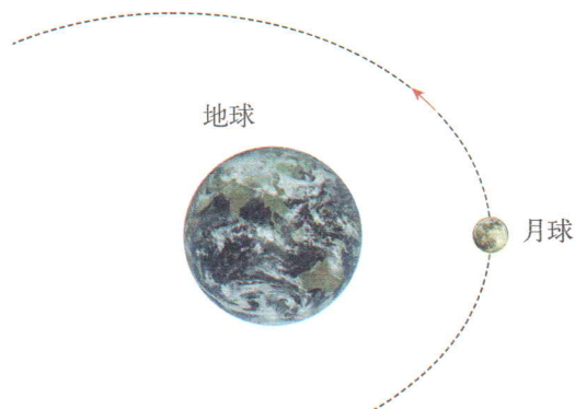
(e) 月球绕着地球转动
