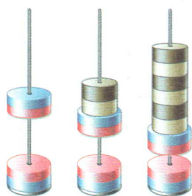
(c) 同名磁极相斥使磁环悬浮
