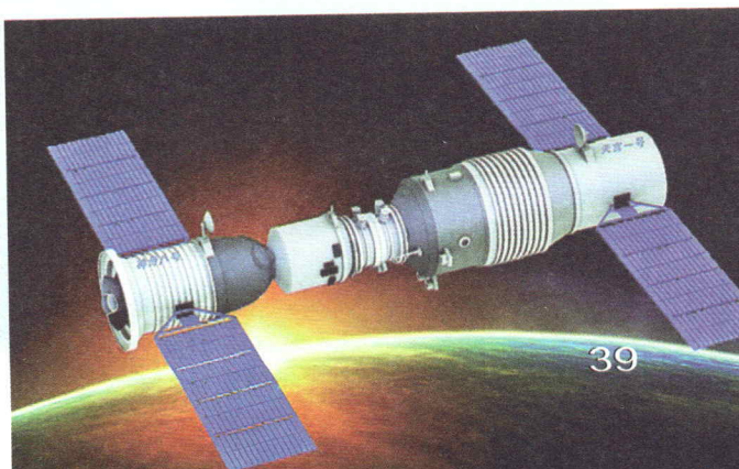
图7-3 “神舟八号”和“天宫一号”对接示意图
