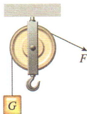
图6-56 斜拉重物的分析
